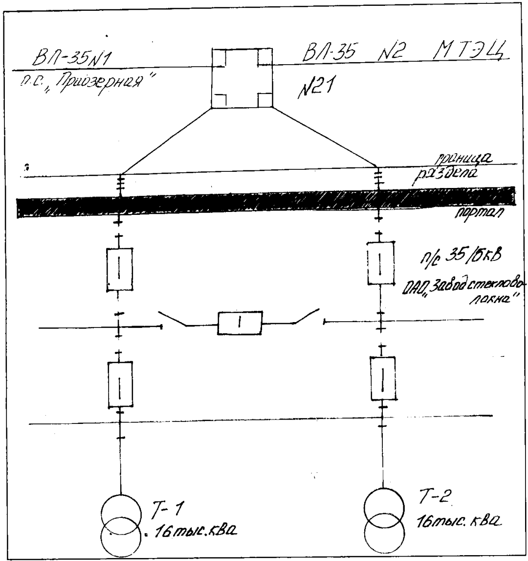
Схема сопряжения сетей:
